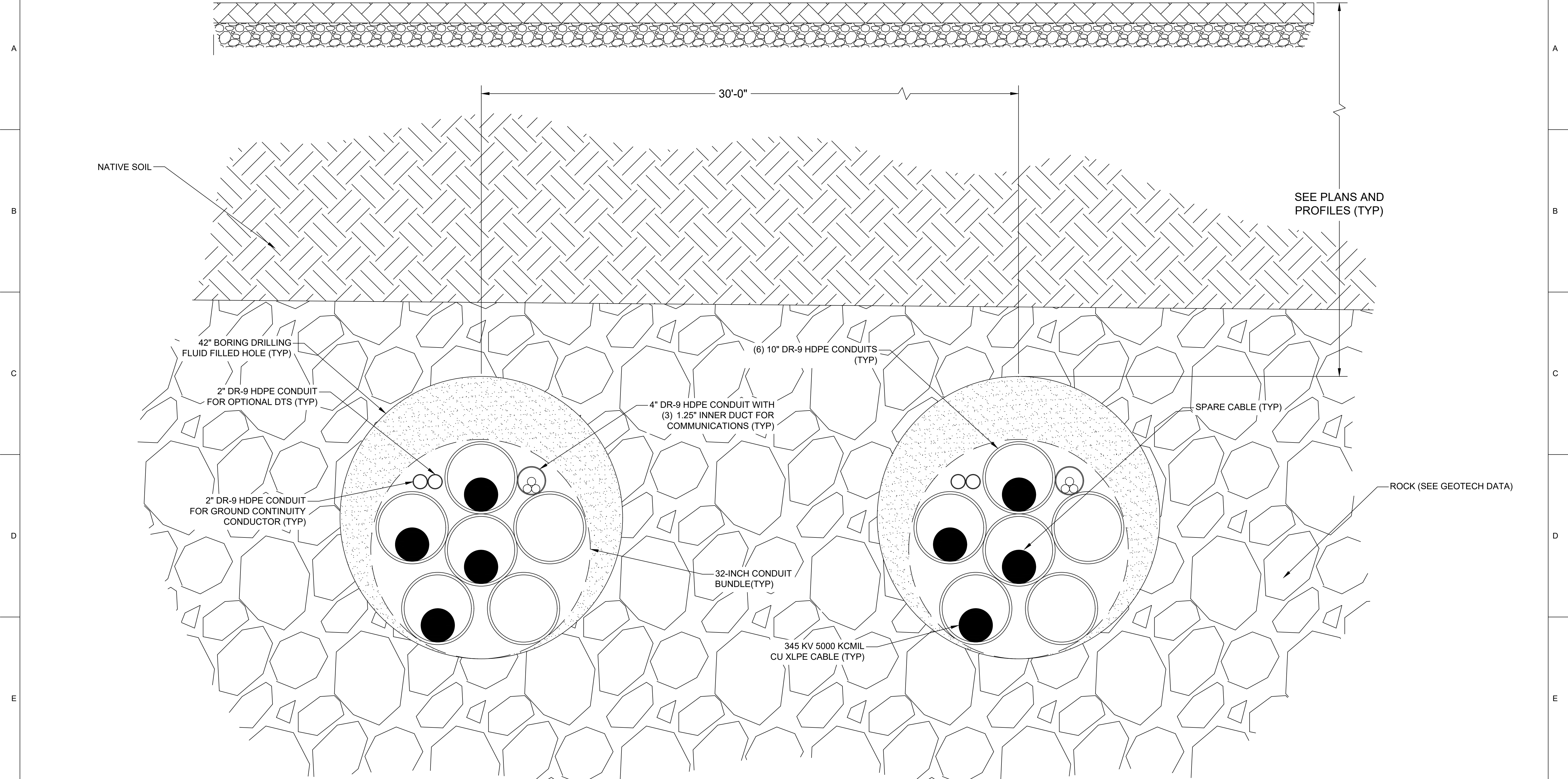
DETAIL BOREHOLE (N.T.S)
